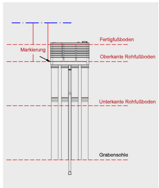
Mehrspartenhauseinführung
